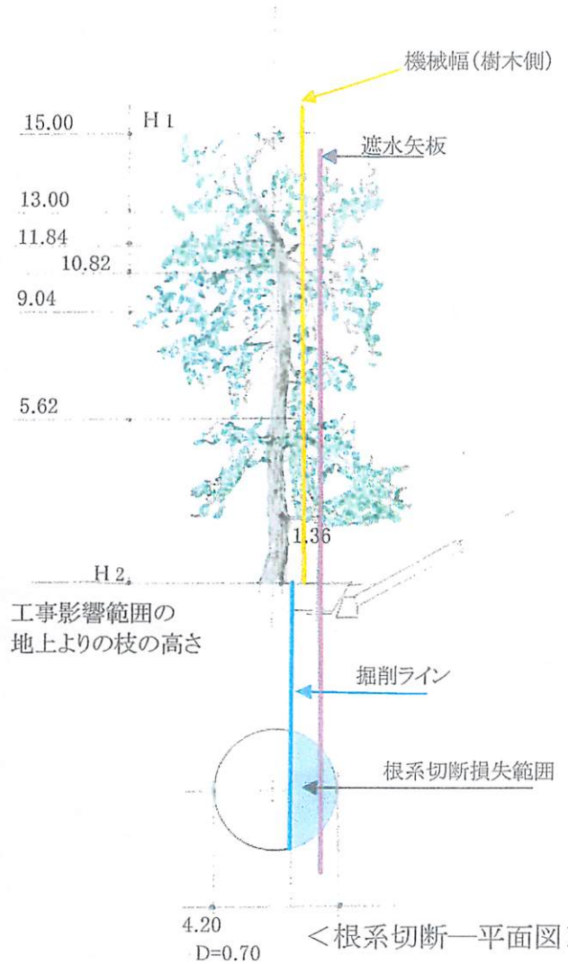
<作業見取図—立面図>
